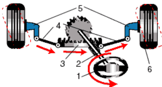
Рис. 48 Схема рулевого управления с механизмом типа «шестерня-рейка»
