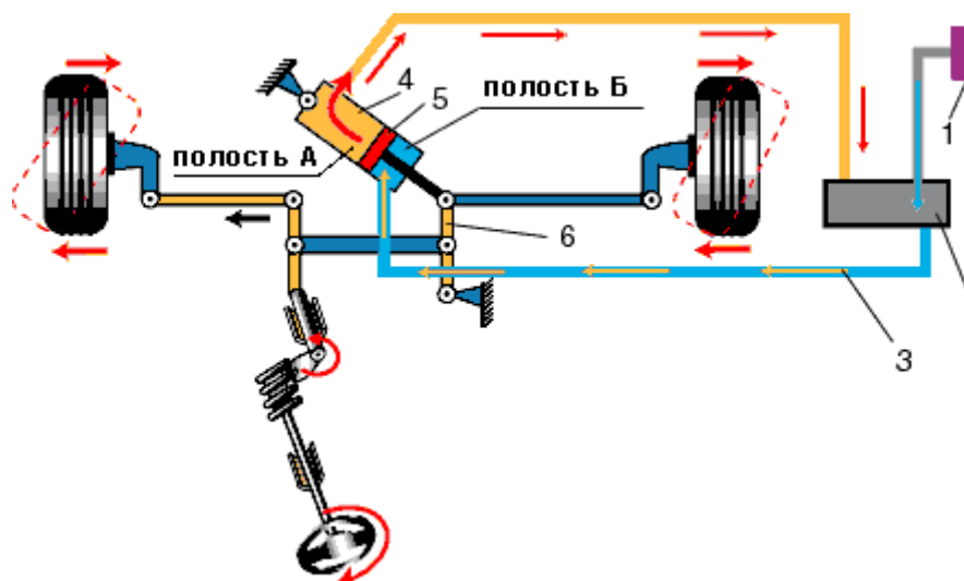
Рис. 49 Схема гидроусилителя рулевого управления 1 - насос усилителя; 2 - распределительное устройство; 3 - трубки для подачи масла; 4 - силовой цилиндр усилителя; 5 - поршень усилителя со штоком; 6 - маятниковый рычаг; 7 - емкость для масла
